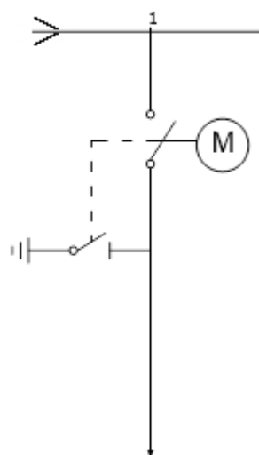
Fig. 1 Schema monofilară
